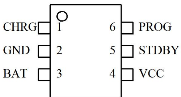
YL4056H、SOT23-6
