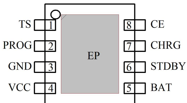
YL4056H、PDFN8(3*3)
