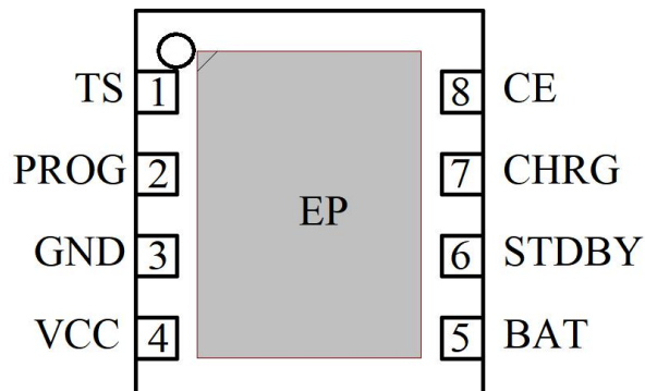
YL4056H、DFN8(3*3)
