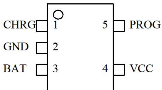
YL4056H、SOT23-5
